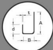
Perfil Jota
