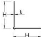
Esquinero
